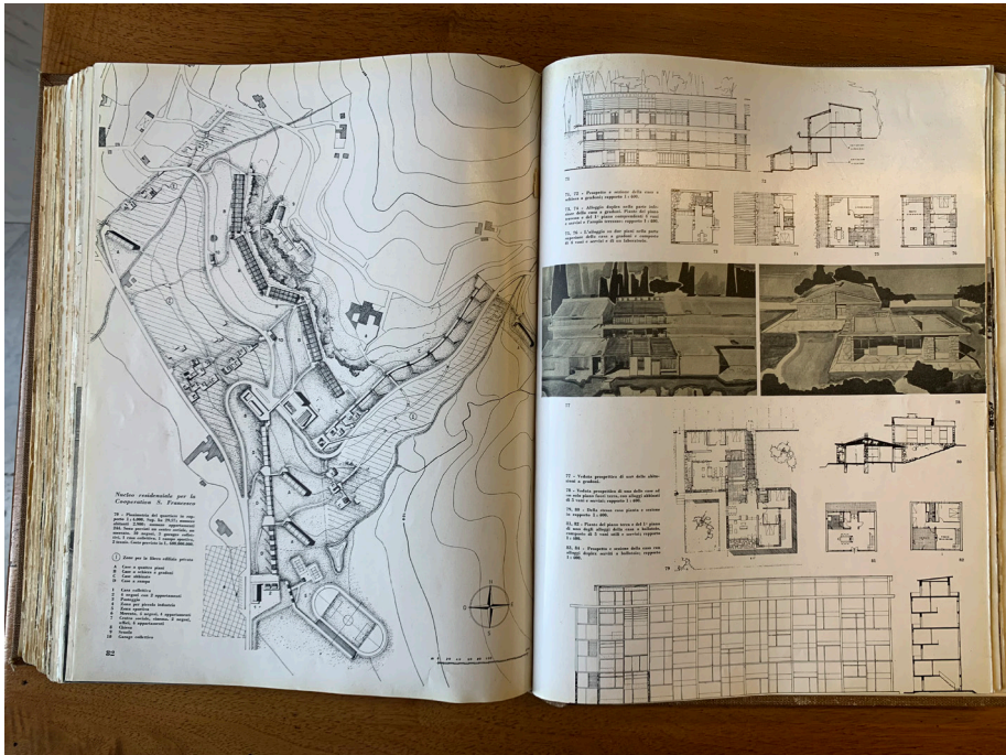
16. Villaggio residenziale per la cooperativa «S. Francesco», in un terreno di circa 30 ha presso Quinto e destinato a 2900 abitanti. Progettato da Danilo Santi e Leonardo Savioli, in relazione a quanto previsto dal recente Piano Regolatore, viene pubblicato nel 1954 sul n. 14 di «Urbanistica»
