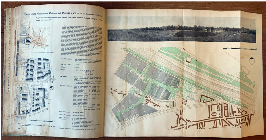
14. Nuova unità residenziale Palazzo dei Diavoli a Firenze. Realizzazione INA Casa. Progetto urbanistico degli ingegneri Burci, Giuntoli, Poggi e degli architetti Pastorini, Pellegrini e Tiezzi. Dicembre 1950 - febbraio 1951, presentato sul n.7 di «Urbanistica» del 1951
