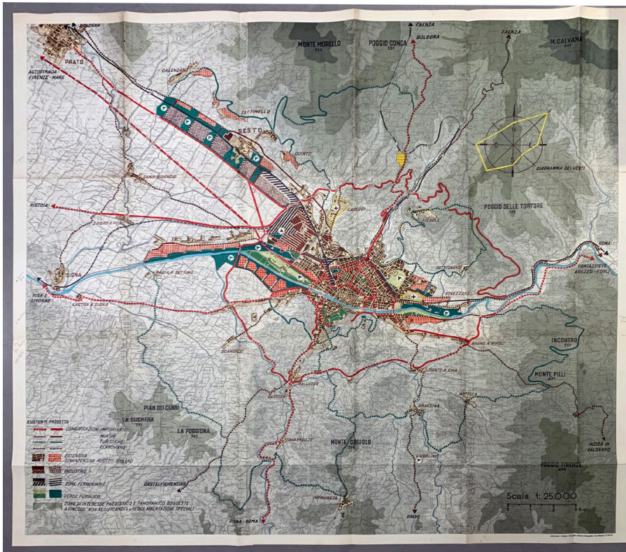
15. Una delle grandi tavole allegate a Relazione al Piano Regolatore Generale di Firenze del 1951 . Si possono notare i percorsi di circonvallazione a nord e a sud della città; in alto a sinistra, verso Prato la fascia destinata agli insediamenti industriali e, in corrispondenza di Quinto, Settimello e Calenzano, zone destinate alla residenza. Altre zone di espansione residenziale si trovano sulla riva sinistra e destra dell'Arno, verso levante a Rovizzano e Villamagna e a ponente, in corrispondenza dell'Isolotto e a nord di Badia a Settimo sull'altra riva del fiume
