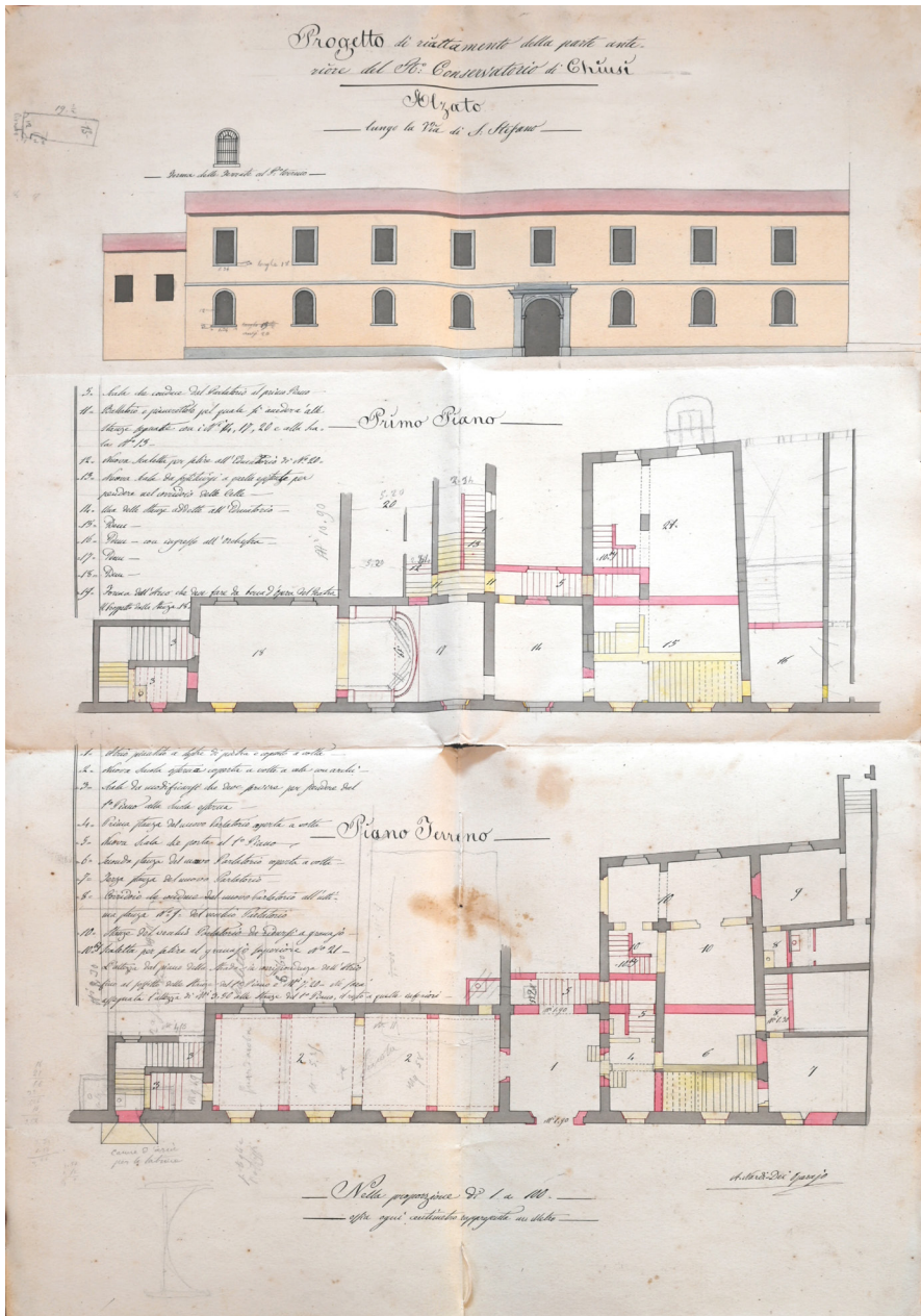
Secondo progetto redatto dal prof. Angiolo Nardi Dei negli anni che vanno dal 1872 al 1876 denominato: "Progetto di riattamento della parte anteriore del R. Conservatorio di S. Stefano di Chiusi" dove sono riportati il prospetto lungo via S. Stefano e le piante del piano primo e terreno della porzione dell'edificio interessate dai lavori. (Archivio Storico Comunale Chiusi)
